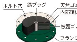
錫プラグ入り積層ゴム支承
