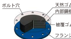
天然ゴム系積層ゴム支承
